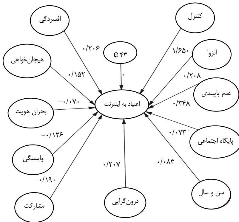
نمودار ۱. معادله ساختاری
